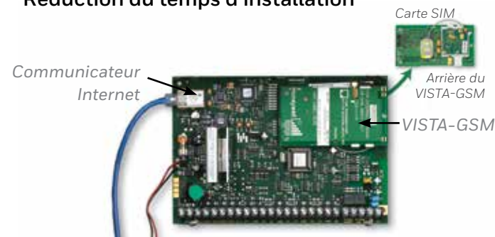
Illustration d'un panneau VISTA-21iP avec radio GSM facultative encliquetable
