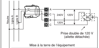
Dia. 2 Bipolaire à trois fils 120/240 V c.a.
