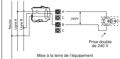
Dia. 1 Bipolaire à deux fils 120/240 V c.a.
