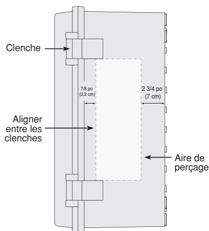
Figure 5 Section de découpage (grosses et très grosses UMM)
