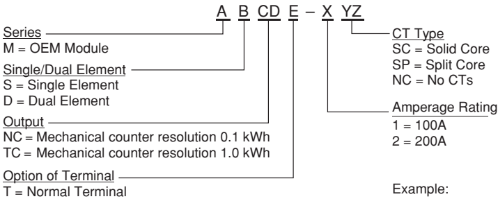
Figure 2 - Mini Meter Model Number Format
