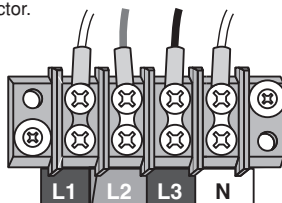
Figura 7 - Bloque de Terminales de Voltaje
