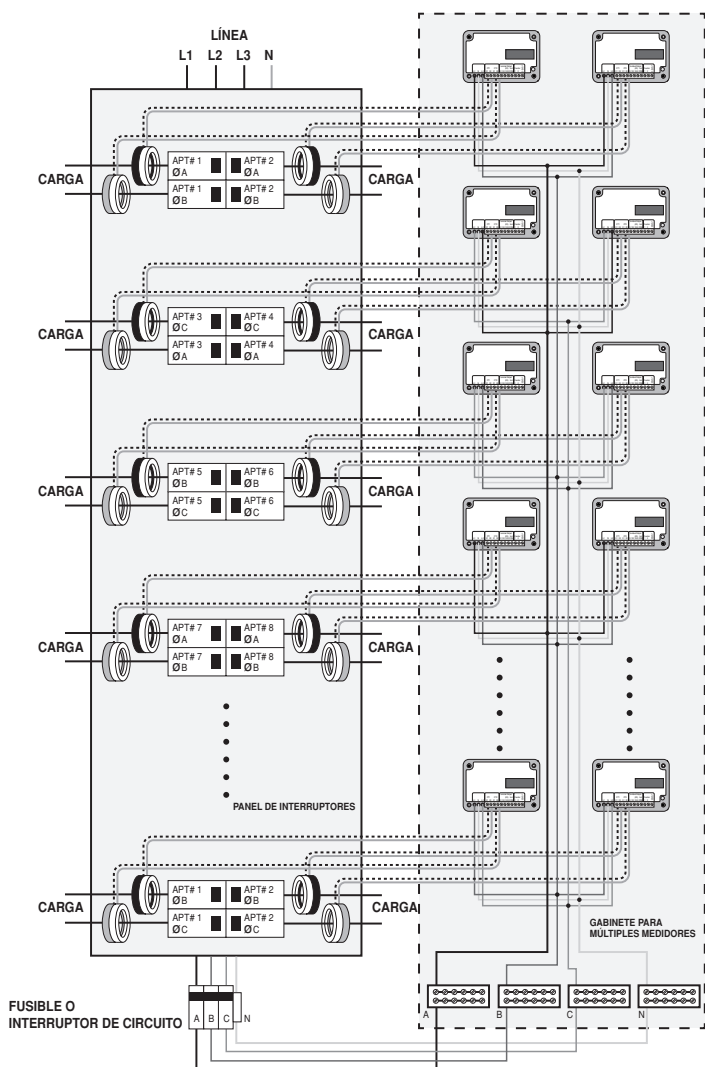
Figura 12: Diagrama de conexión para 3 Fases y 4 Cables
