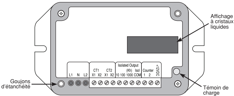
Figure 4 - Connexions et affichage des minicompteurs
