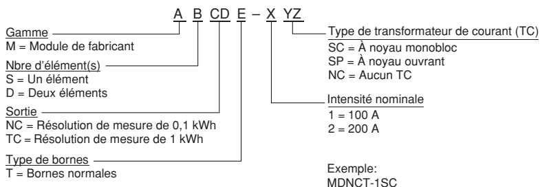
Figure 2 - Composition des numéros de modèle des minicompteurs
