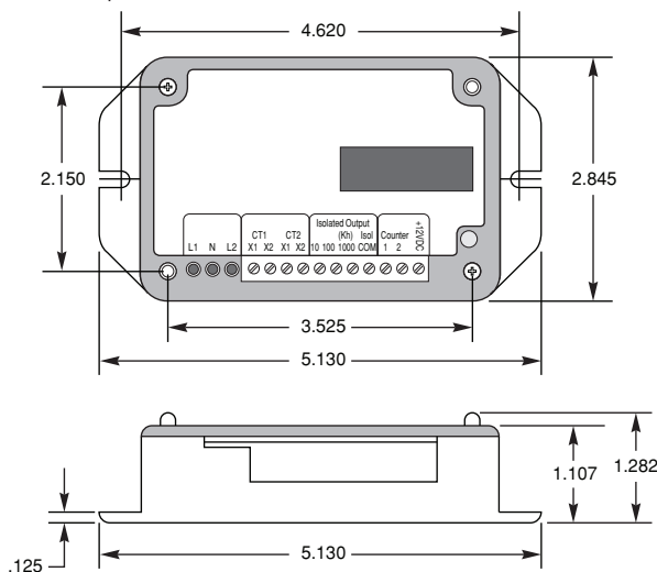
Figure 1 - Dimensions externes d'un minicompteur
