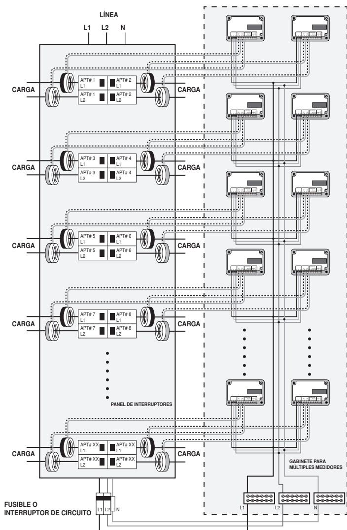
Figura 11: Diagrama de conexión de 2 fases (fase dividida), 3 cables
