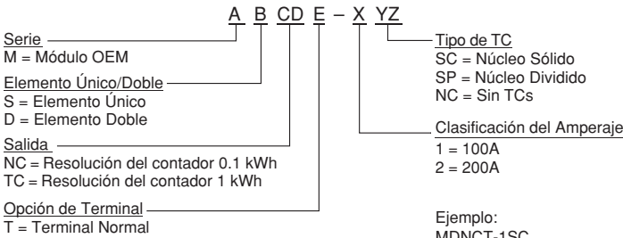
Figura 2 - Formato de Número de Modelo de Mini Medidor
