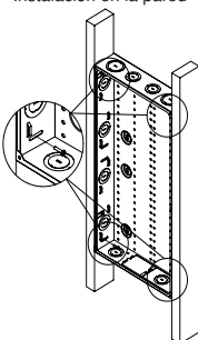
Instalación en la pared
