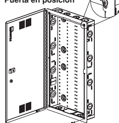
Puerta en posición
