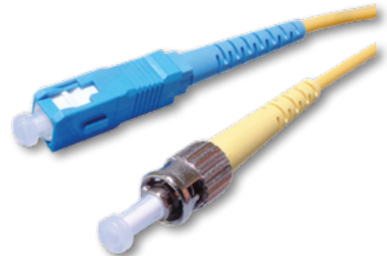
Simplex SC-ST-SM
