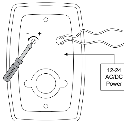
CM-AF141SO Wiring
