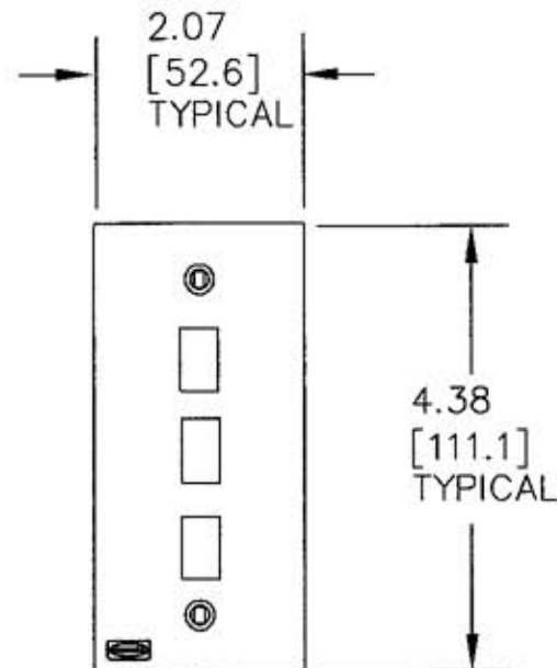
KP2163/KP2163AL/, KP2163GY JACK-JACK-JACK
