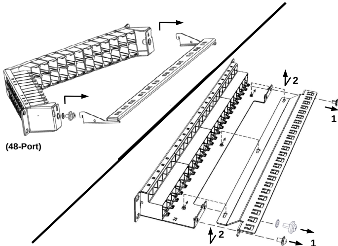
48-Port angled
