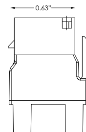
Cat5e 180° Keystone
