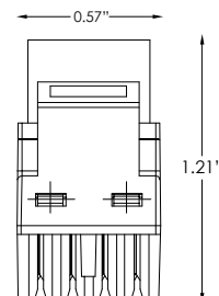
Cat5e 180° Keystone
